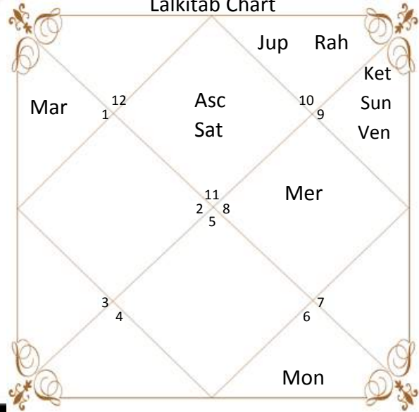
Lalkitab Chart
